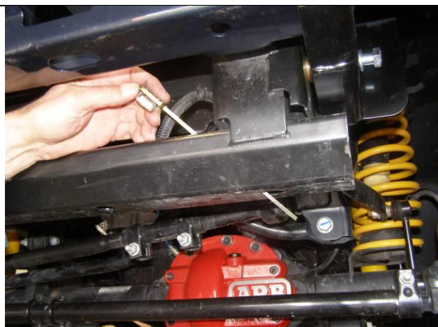
LHS Shown
